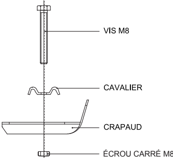
ATTACHE AVEC CAVALIER
