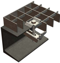
PRINCIPE DE POSE
