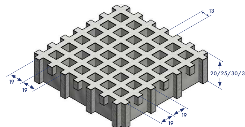
MAILLE DE SÉCURITÉ 19 X 19
