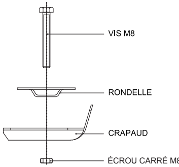
ATTACHE AVEC RONDELLE
