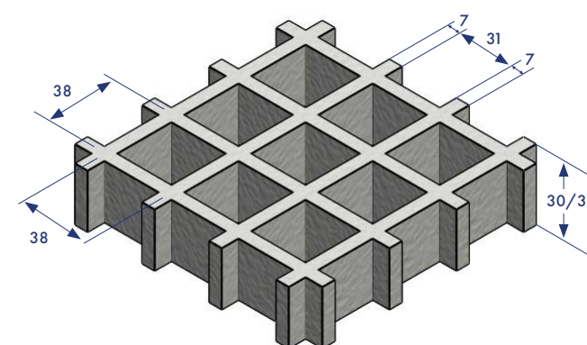
MAILLE STANDARD 38 X 38
